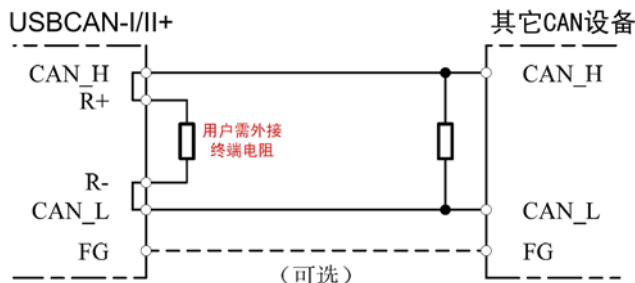
图2.2 USBCAN与其他CAN设备的连接
