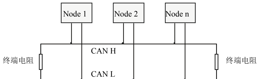
图2.1 CAN-bus网络的拓扑结构
